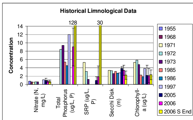
Fig. 26. Historical lake data.
