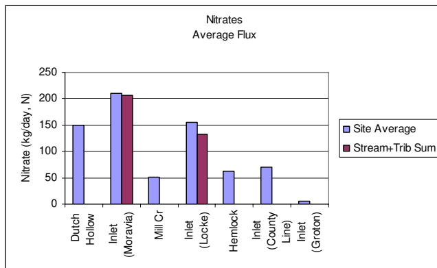
Fig. 24. Site averaged nitrate flux.
